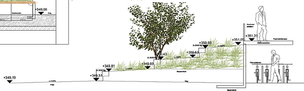
Systemschnitt Hochbeet/ Feuerwehrterrasse (M:1:25)
