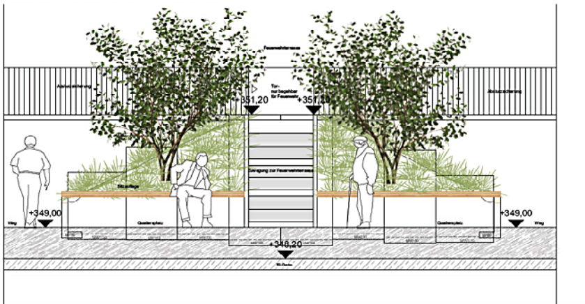
Systemansicht Hochbeet und Feuerwehrterrasse (M:1:25)
